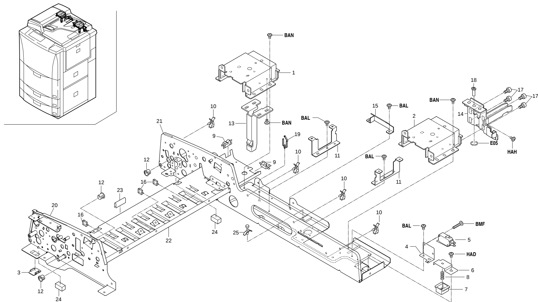
FIG.38 FRAMES (DF)
