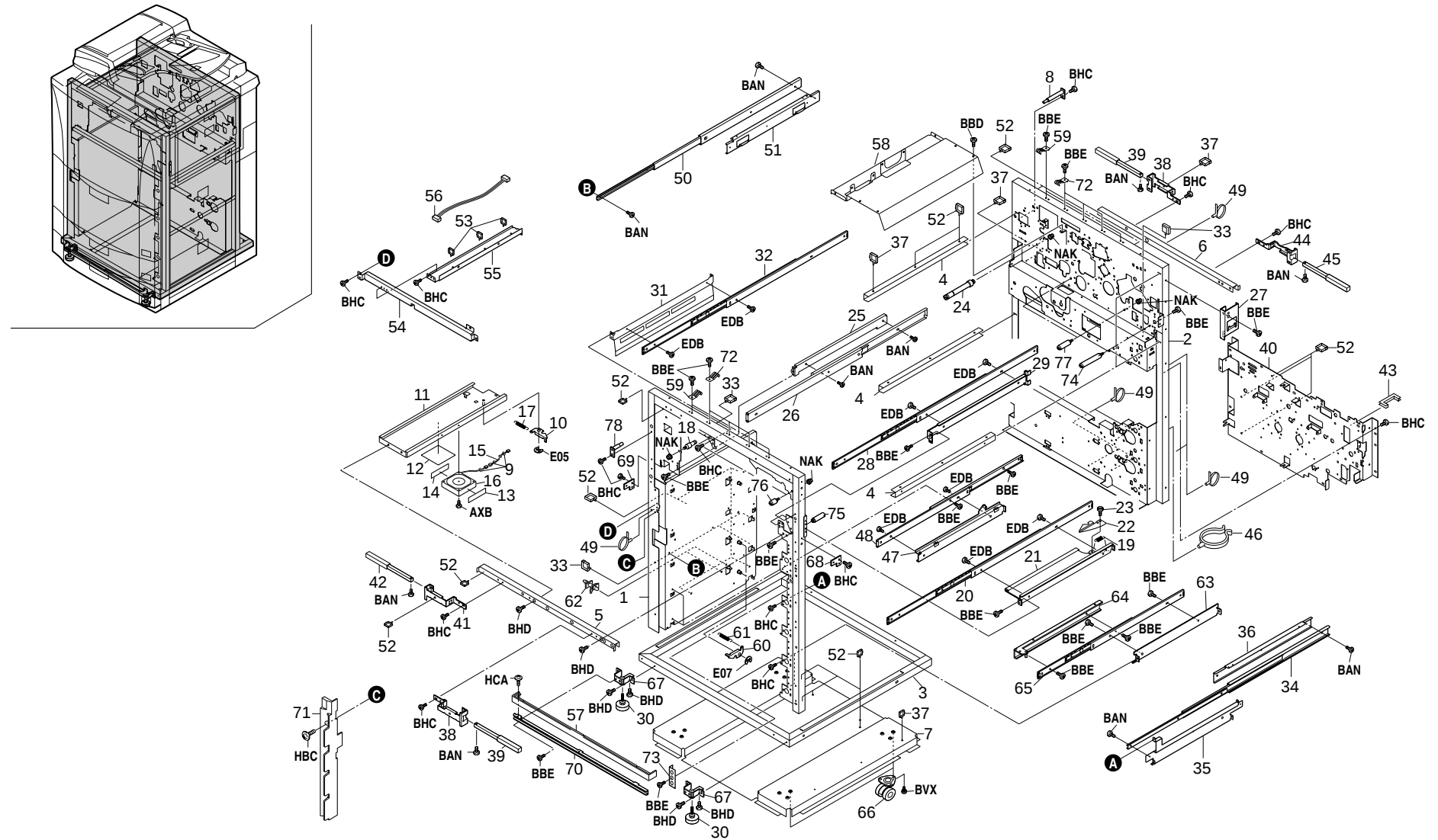
FIG. 2 FRAMES
