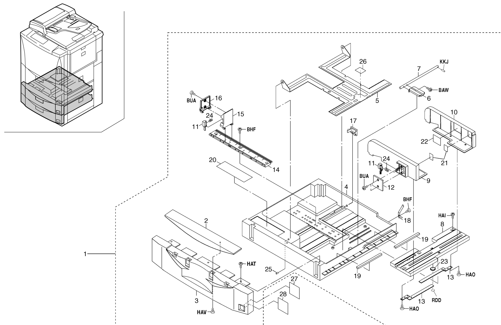
FIG. 3 CASSETTE(230/240V)
