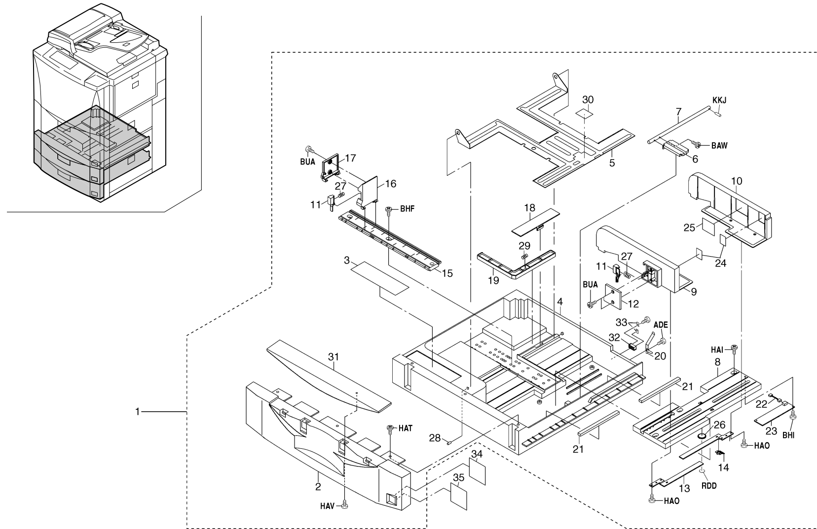
FIG. 3 CASSETTE(120V)
