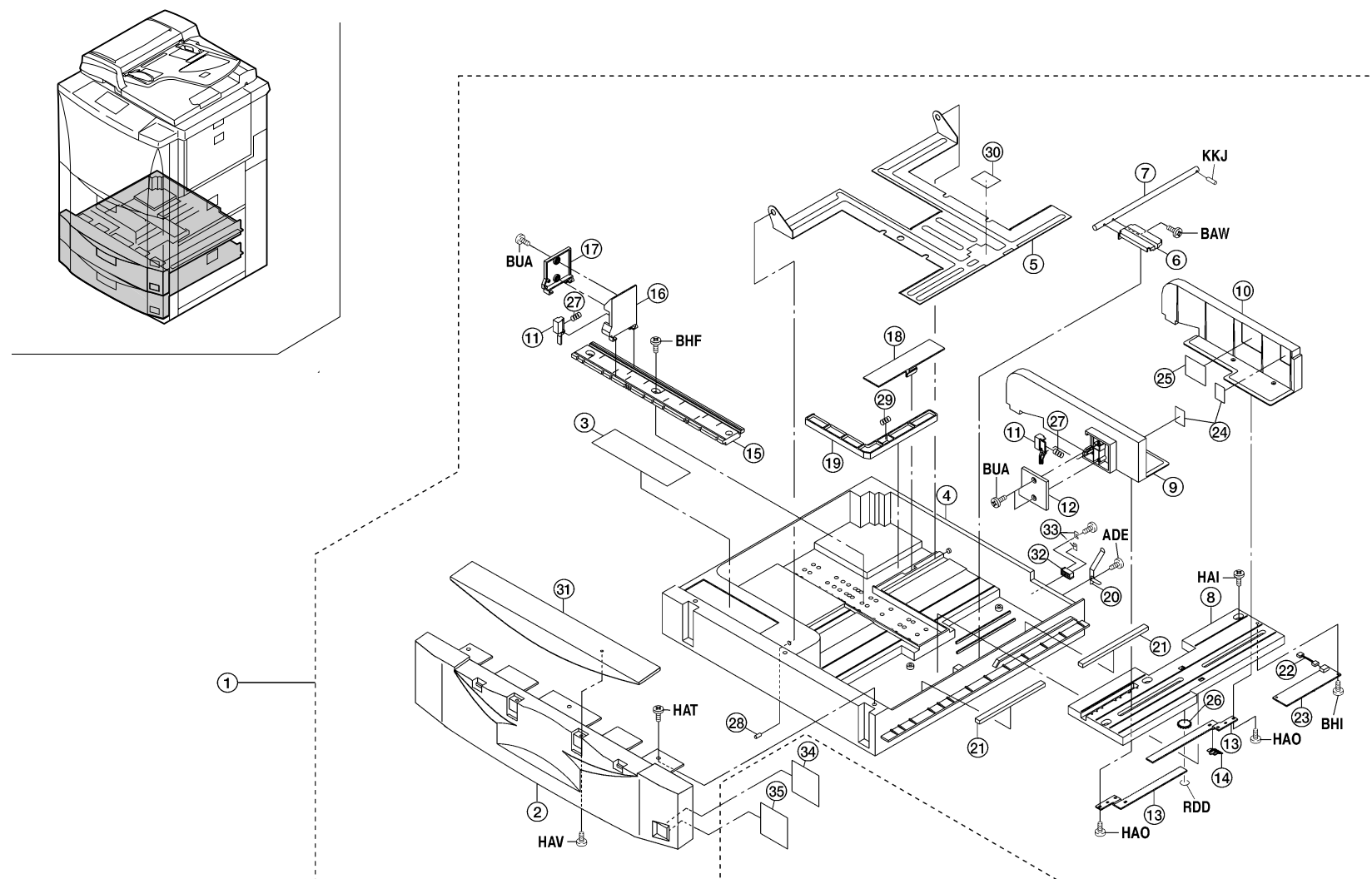
FIG. 3 CASSETTE(120V)
