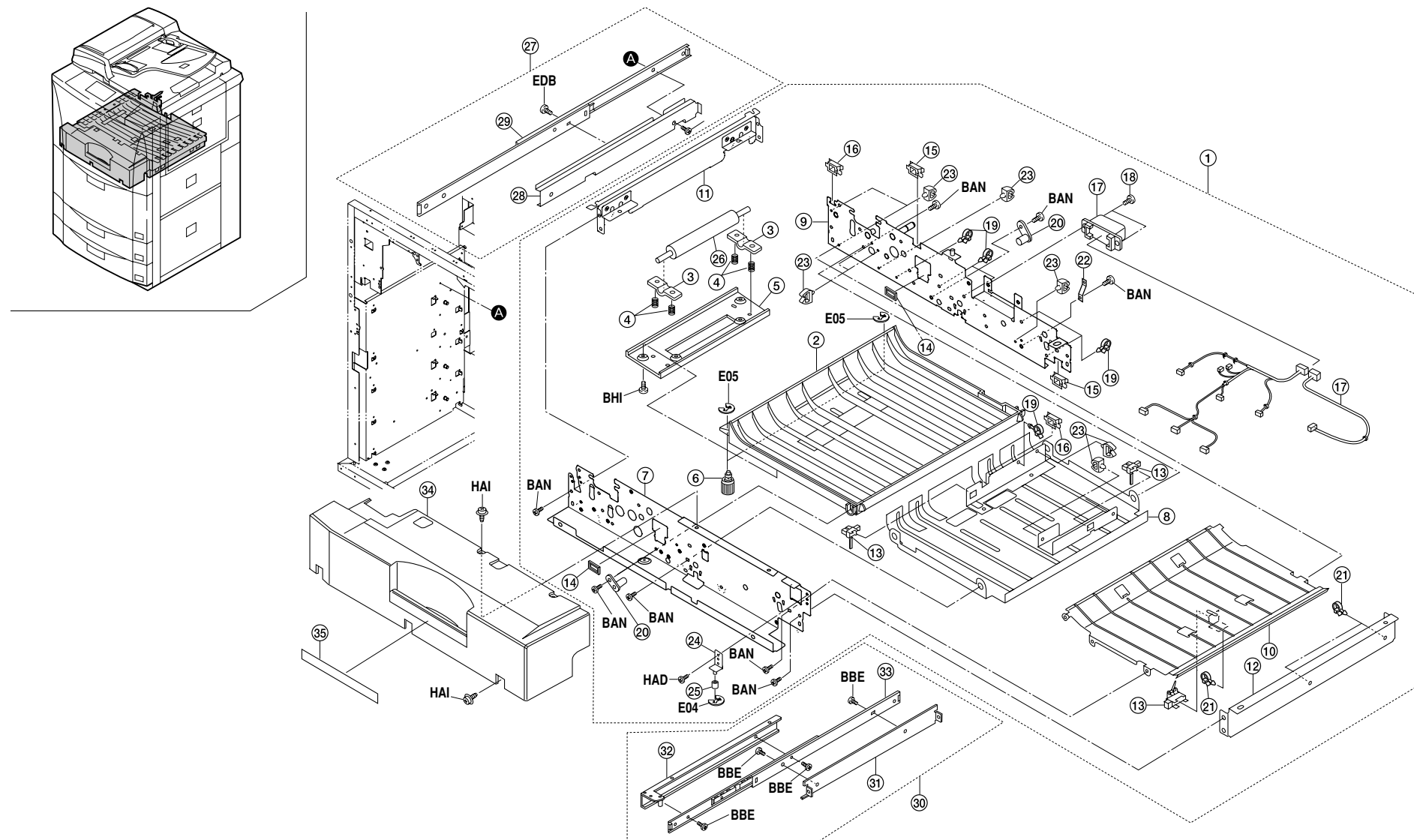
FIG.27 DUPLEX UNIT I
