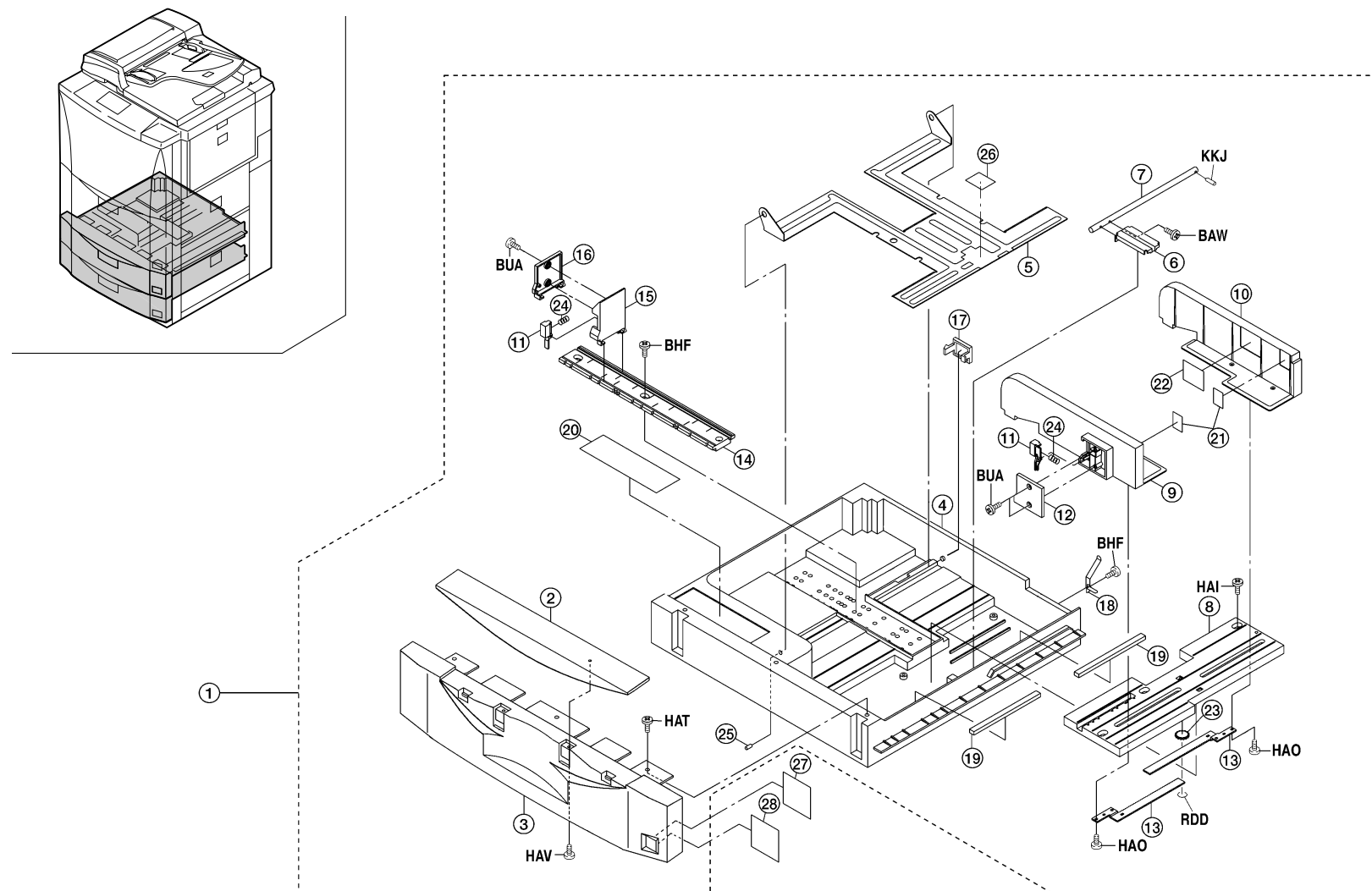
FIG. 3 CASSETTE(230/240V)
