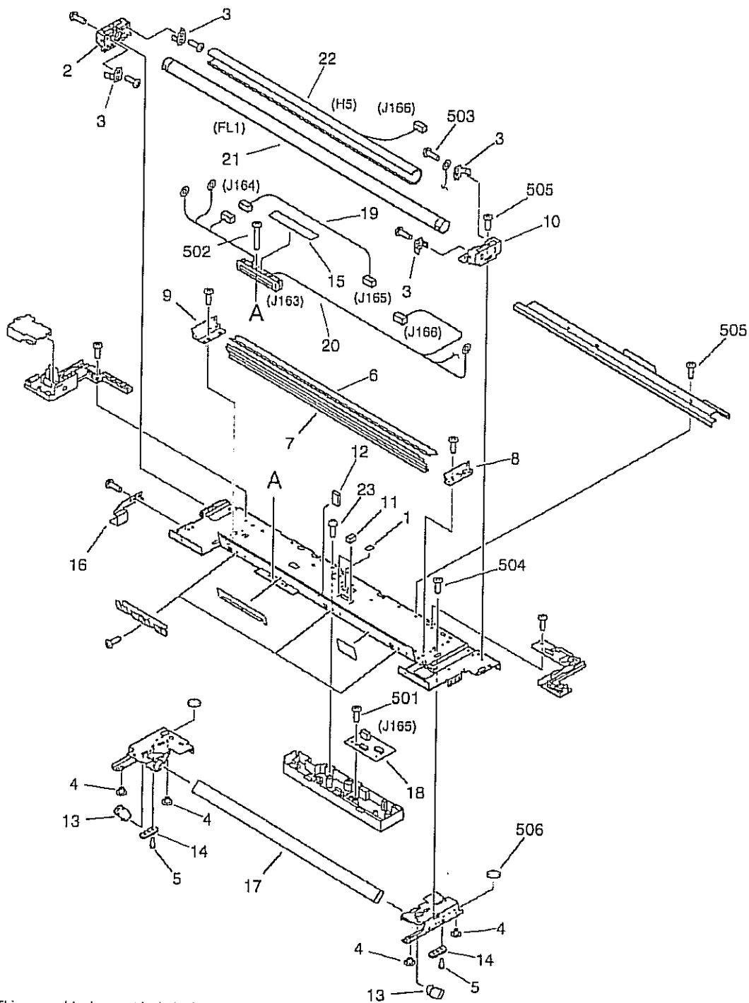
FIGURE 420 MIRROR ASSEMBLY 1 第1ミラー台部
