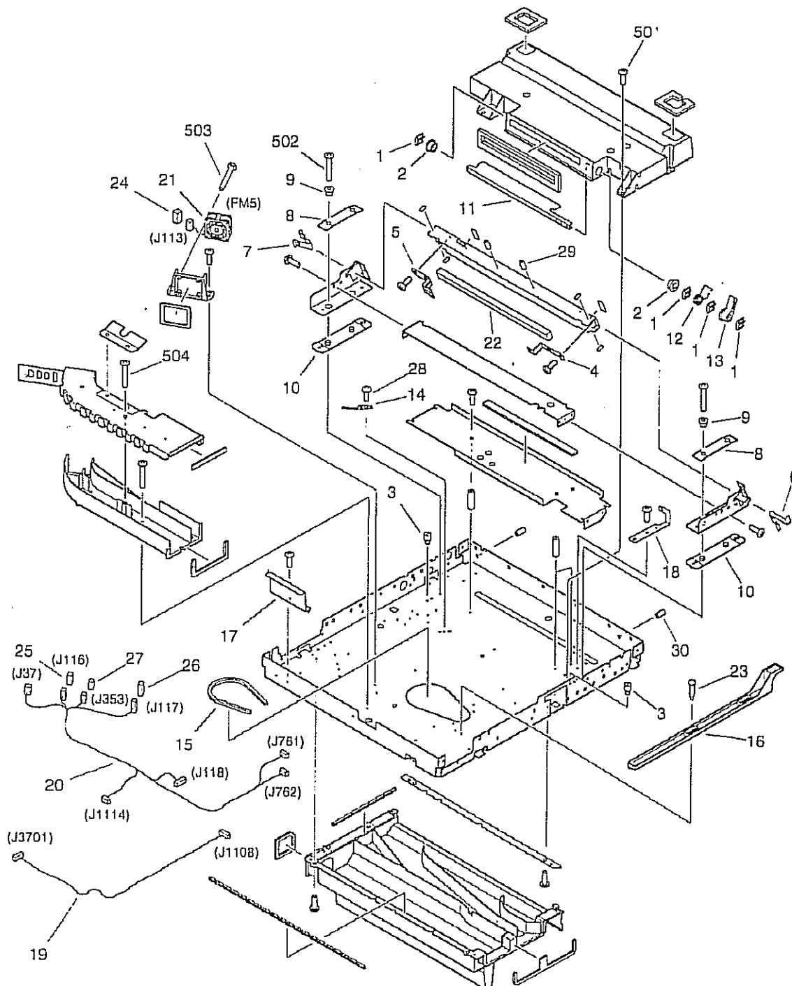
FIGURE 215 SCANNER MOUNT ASSEMBLY スキャナ台部
