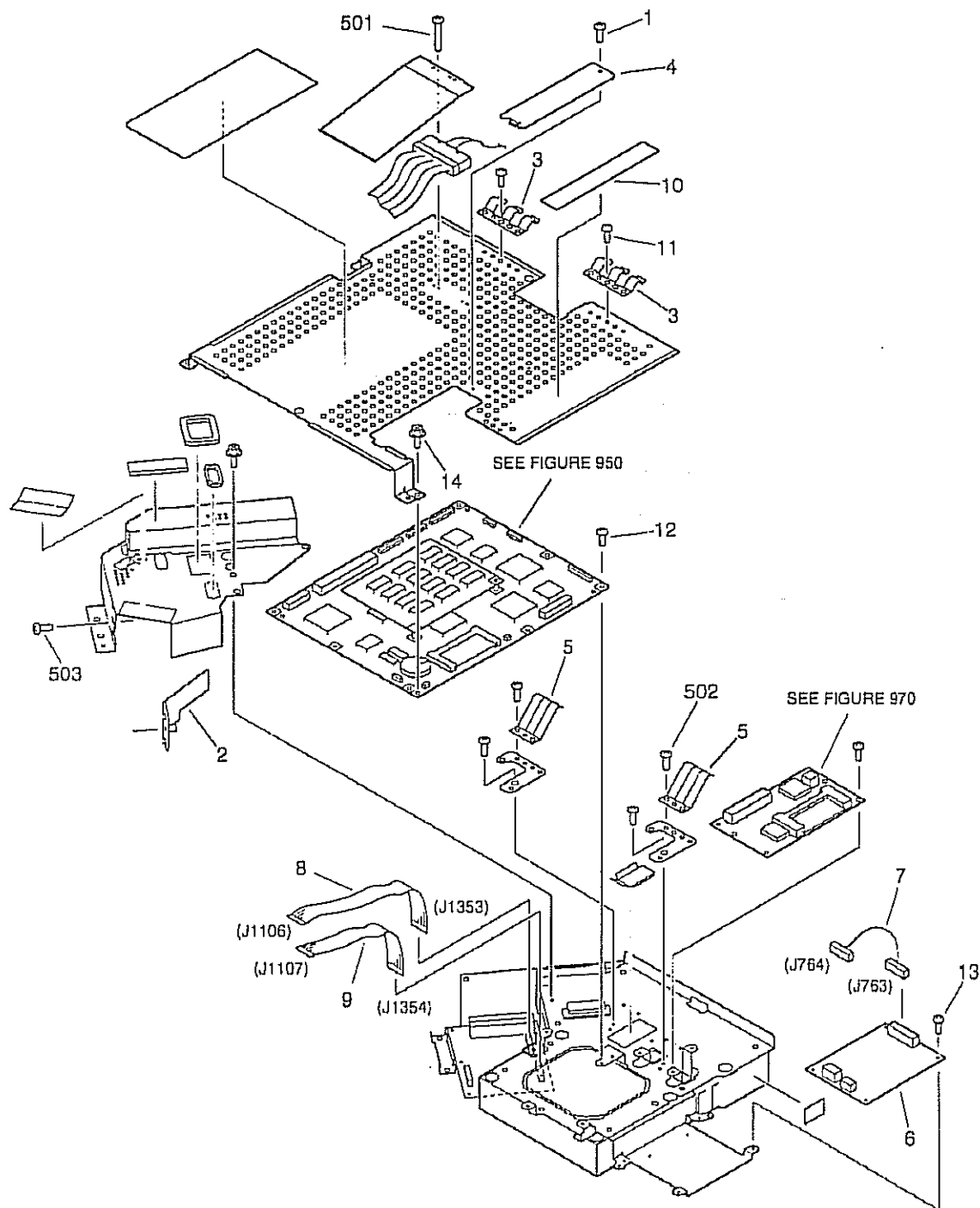
FIGURE 460 SCANNER ASSEMBLY スキャナ部
