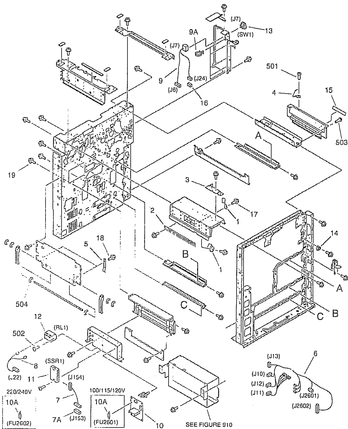
FIGURE 105 INTERNAL COMPONENTS 4 本体機械内部 (4)
