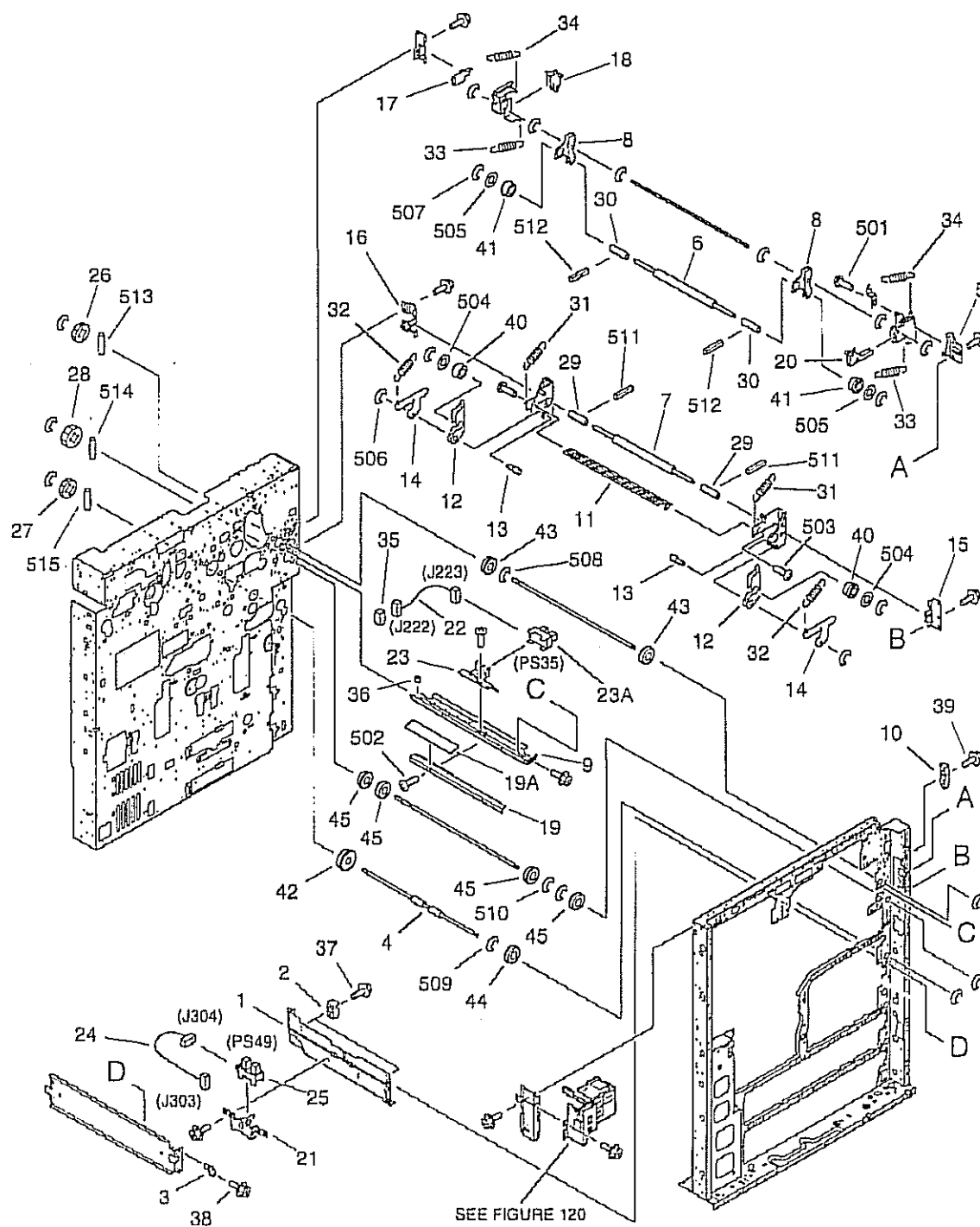
FIGURE 102 INTERNAL COMPONENTS 1 本体機械内部 (1)
