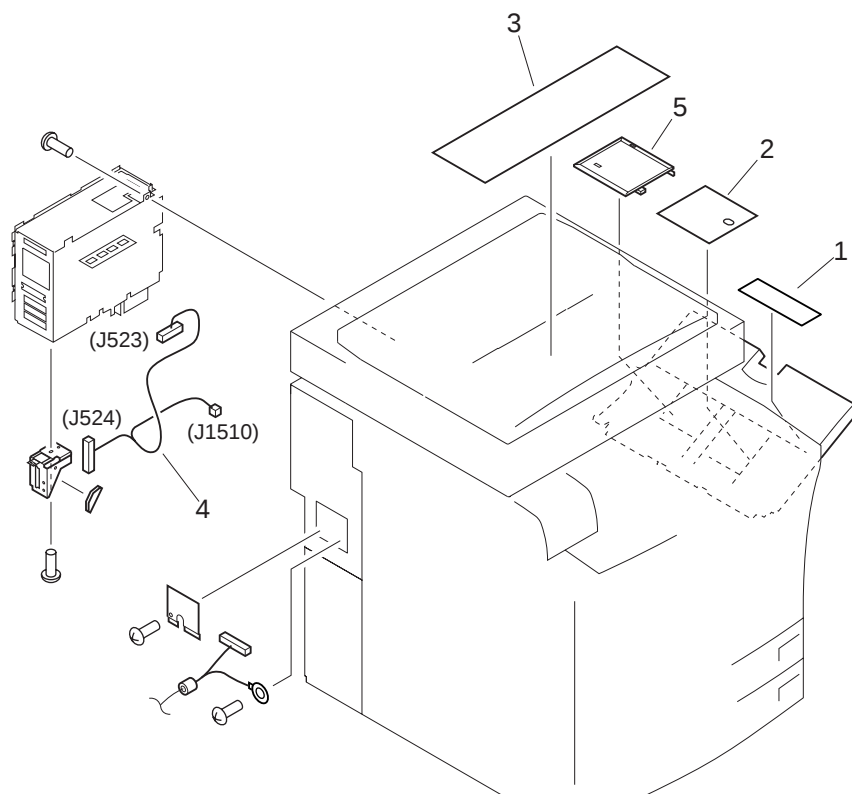
FIGURE Y11 SELF OPERATION KIT (100V) セルフ対応キット (100V)
