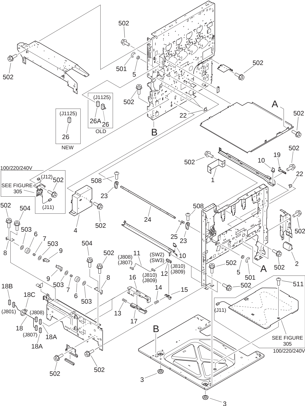
INTERNAL COMPONENTS 1 本体機械内部 (1)
