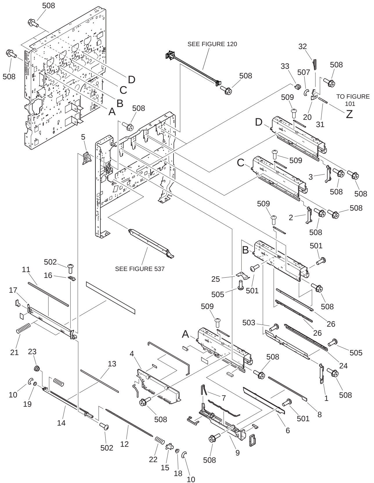
FIGURE 104 INTERNAL COMPONENTS 3 本体機械内部 (3)
