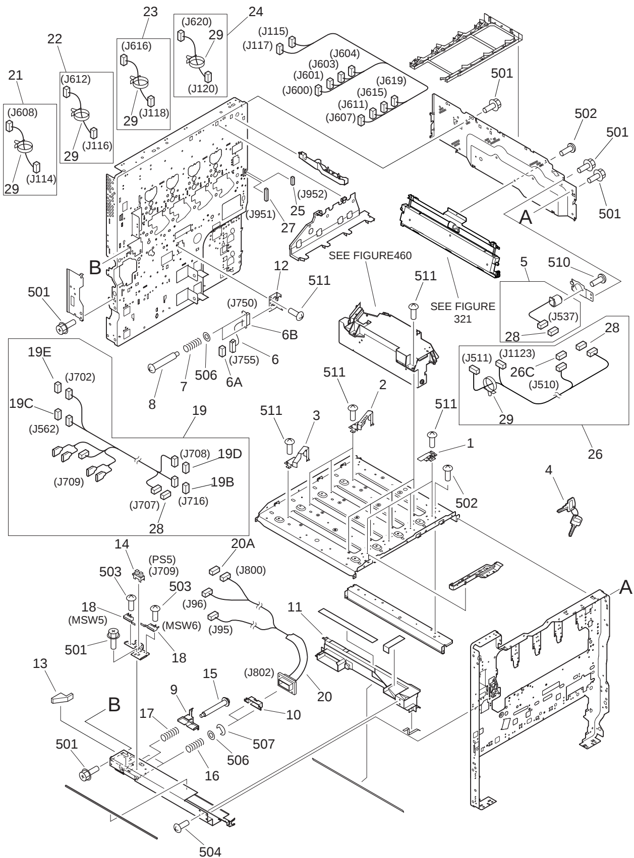
FIGURE 105 INTERNAL COMPONENTS 4 本体機械内部 (4)
