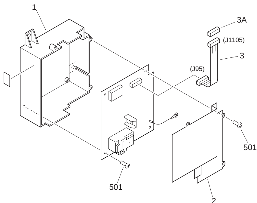
FIGURE 981 2ND. TRANSFER H.V.T. PCB ASSEMBLY 二次転写高圧トランス回路基板
