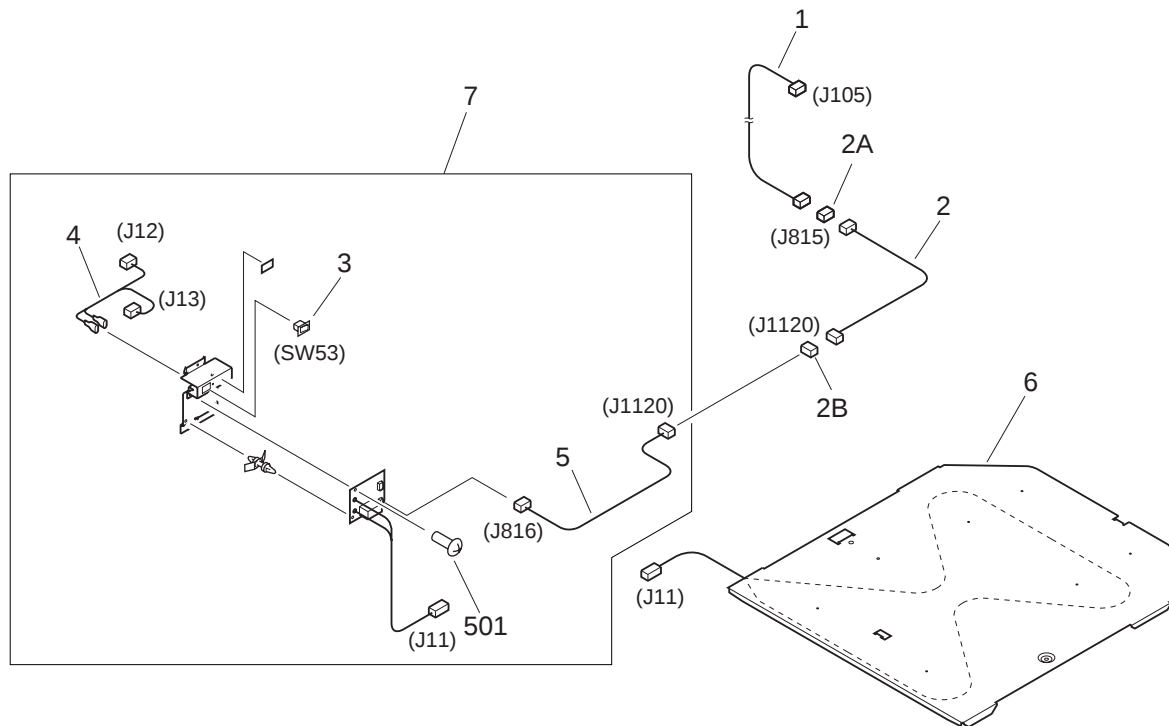
FIGURE 305 CASSETTE HEATER ASSEMBLY (OPTION) カセットヒータ部（オプション）
