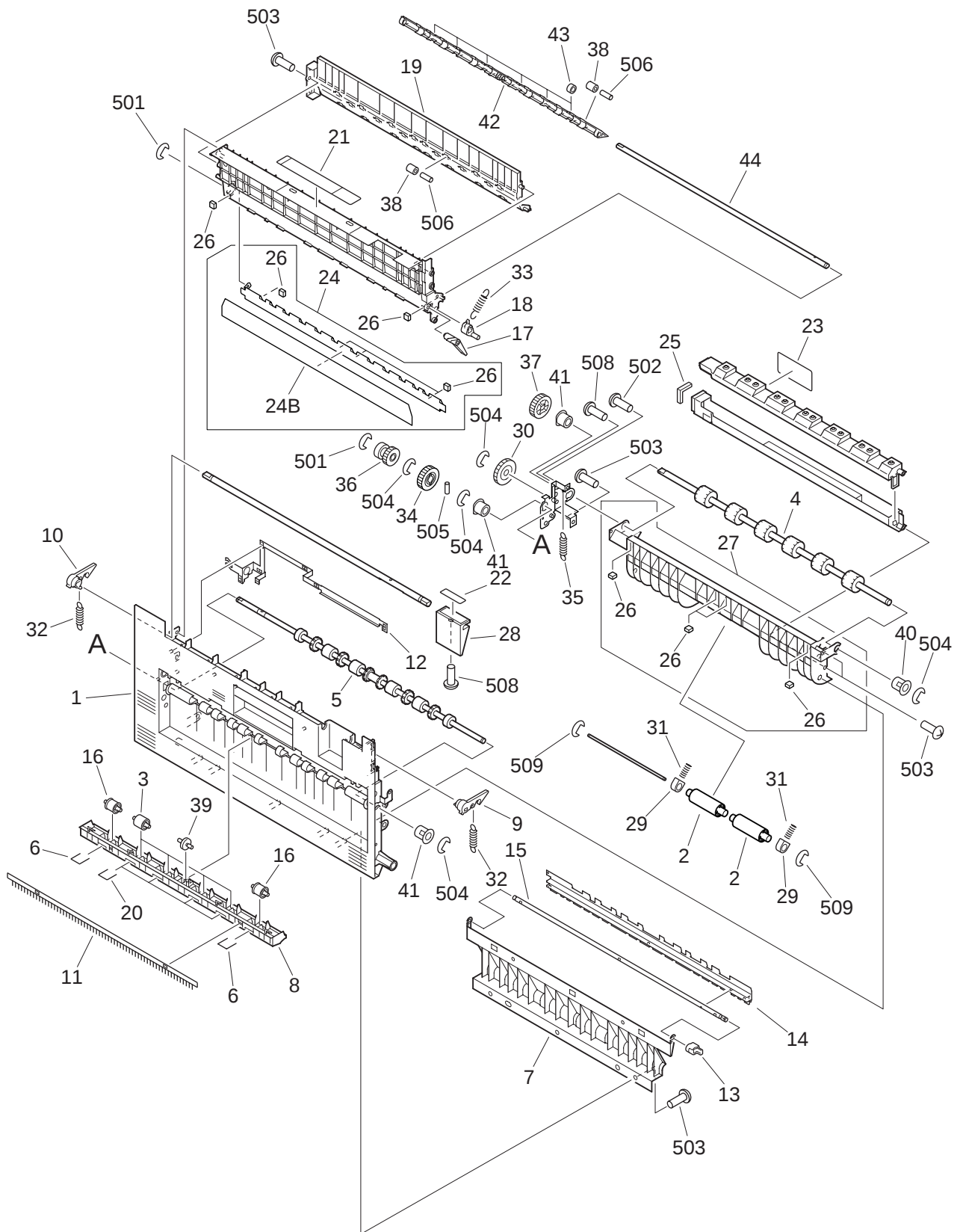
FIGURE 361 EXTERNAL DELIVERY COVER ASS'Y (DUPLEX TYPE) 外排紙開閉カバー部（両面タイプ）
