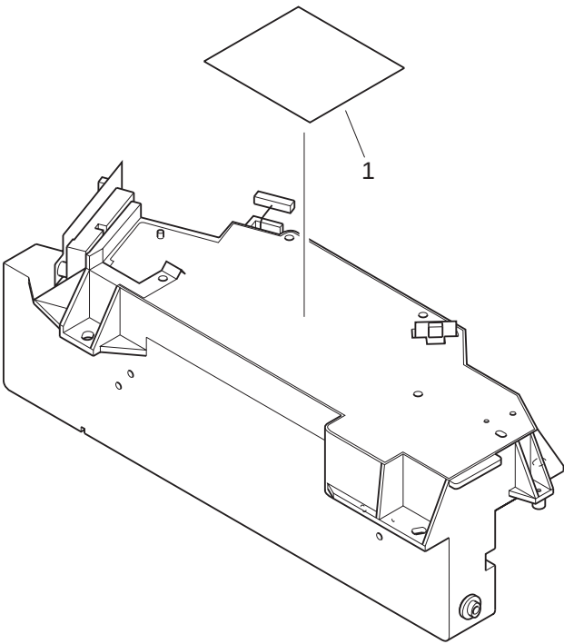
FIGURE 460 LASER UNIT レーザユニット
