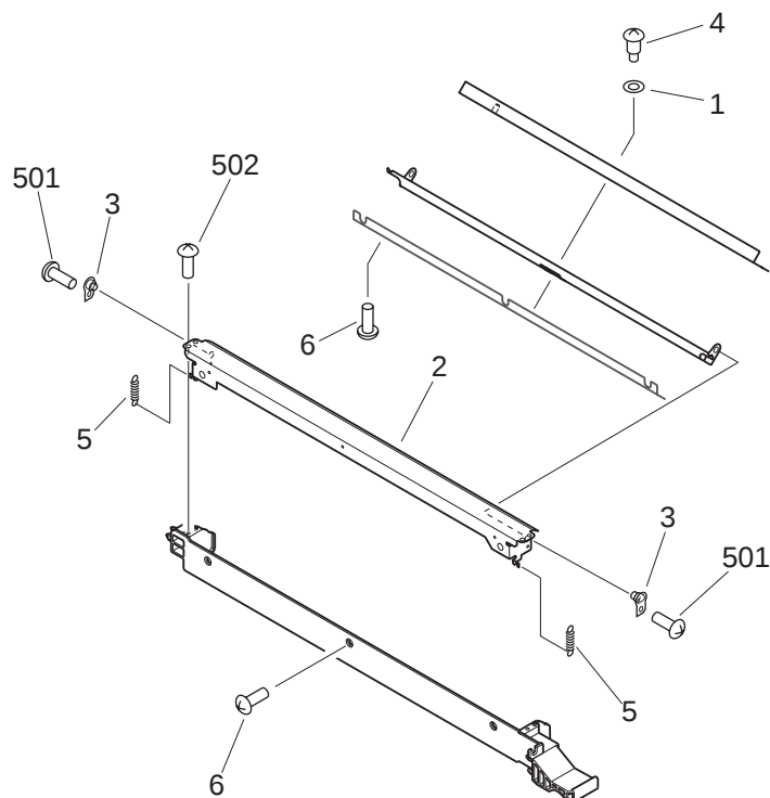
FIGURE 537 TRANSFER CLEANING ASSEMBLY 転写クリーニング部
