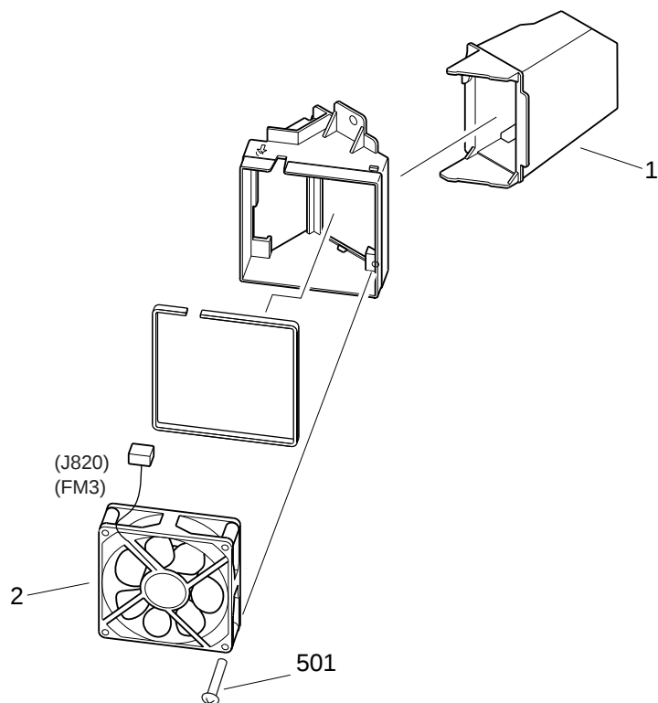
FIGURE 192 MACHINE EXHAUST FAN ASSEMBLY 本体排熱ファン部
