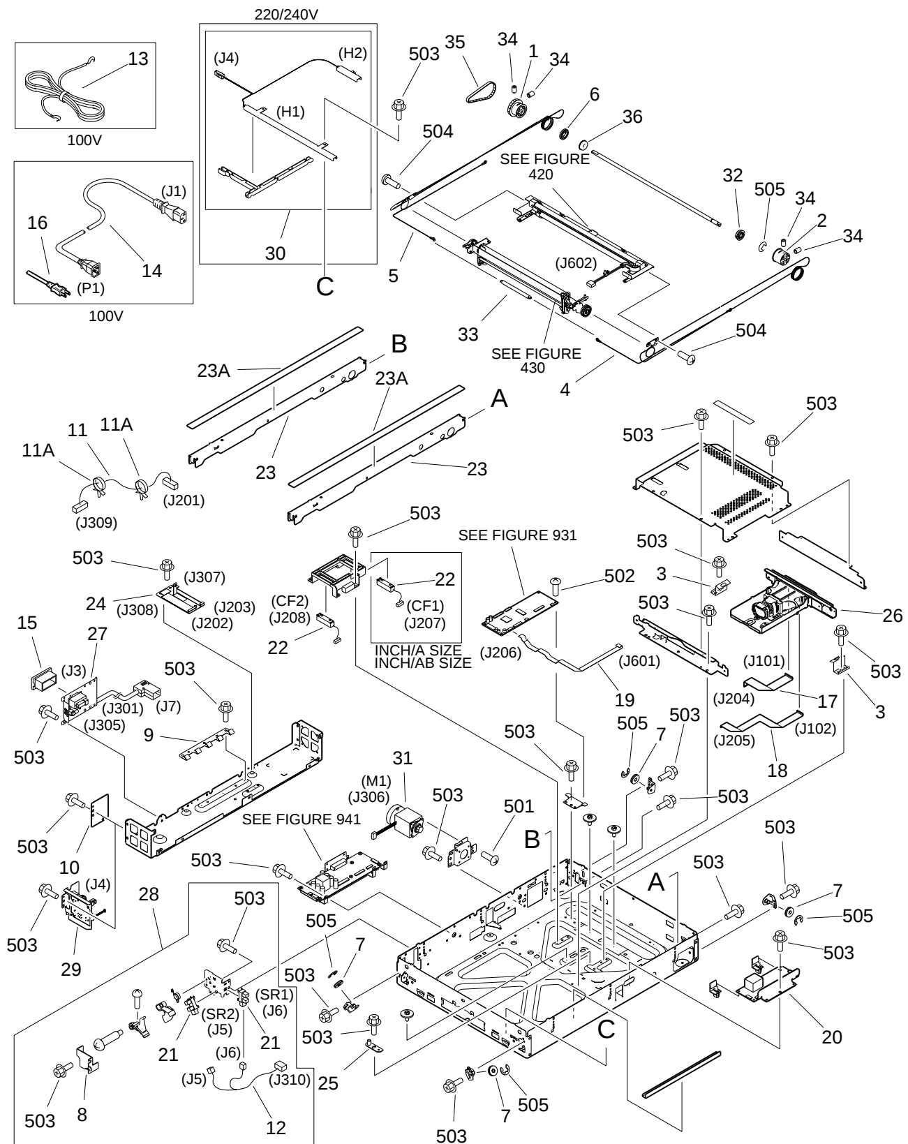
FIGURE 210 READER ASSEMBLY リーダ部
